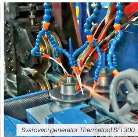
Délka linky 70 m | válcovací rychlost 80 m/min
